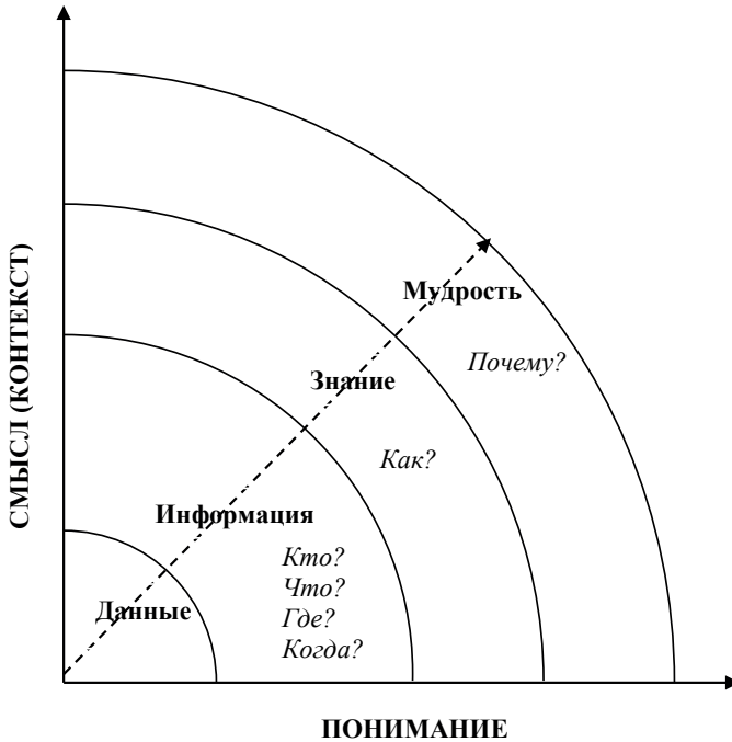
Рисунок 4 – DIKW-модель
